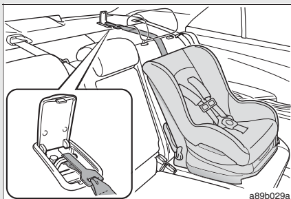
トップテザーアンカー (→P. 99)
