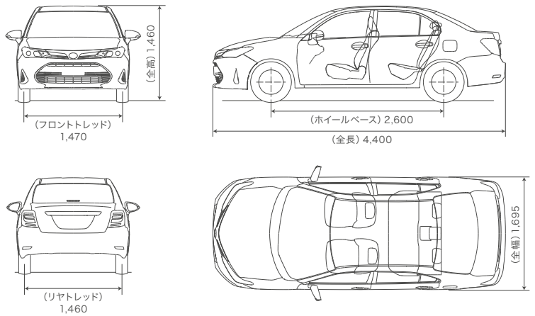
寸法図:トヨタ カローラ アクシオ1.5G(2WD) (単位mm)
