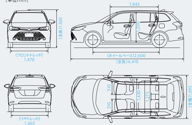
寸法図: トヨタ カローラ フィールダー 1.8S "W×B" (2WD)
