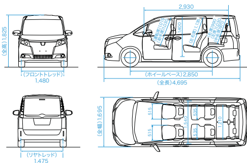
寸法図:トヨタ エスクエア Gi (7人乗り・2WD)
