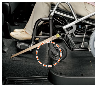
⑥車いすの前輪が車輪止めに到達したら、車いすを止めます。セーフティベルトにより、車いすの前側が固縛されます。 ※写真はメーカーオプションの電動ウインチ装着車です。
