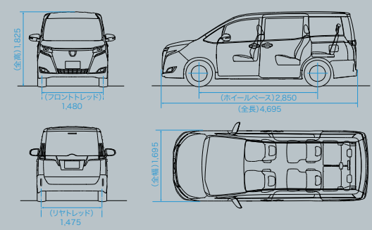
寸法図:トヨタ エスクエア Gi (7人乗り・2WD) 単位:mm
