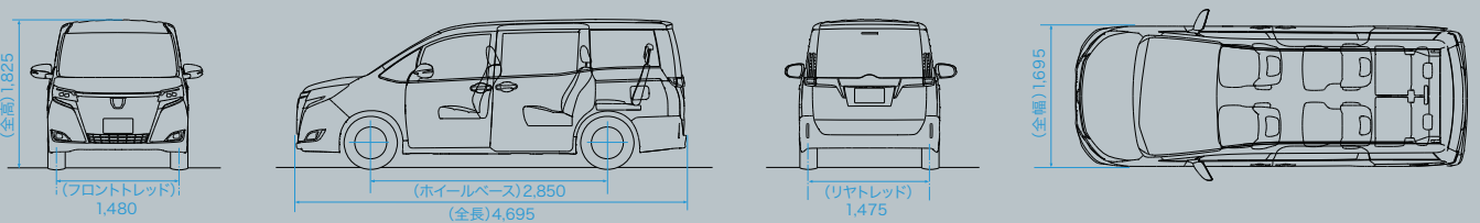
寸法図:トヨタ エスクエアア Gi (7人乗り・2WD) 単位:mm
