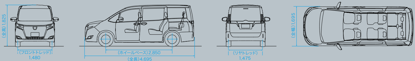
寸法図:トヨタ エスクエア Gi (7人乗り・2WD) 単位:mm
