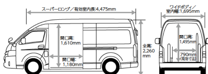
Photo: 車いす仕様車「Dタイプ」2WD-2700ガソリン スーパーロング・ワイドボディ(3BF-TRH223B-VTZYD) ボディカラーはホワイト(058)。専用車いす「ウェルチェア」は販売店装着オプション。汎用車いすは装備に含まれません。
