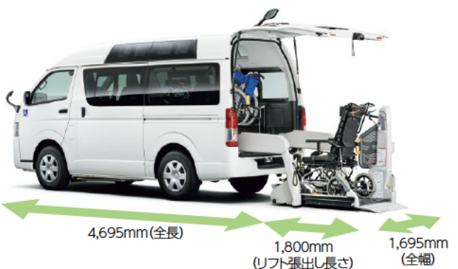
Photo: 車いす仕様車「Aタイプ」ルーフサイドウインドウ装着車 2WD-2000ガソリン ロング・標準ボディ(3BF-TRH200-VTZYAW) ボディカラーはホワイト(058)。大型車いす、汎用車いすは装備に含まれません。
