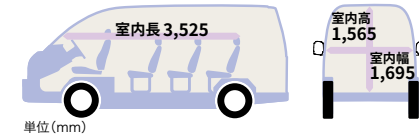
単位(mm)
