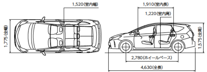
S(5人乗り) フレンドマチック取付用専用車“タイプ I”
