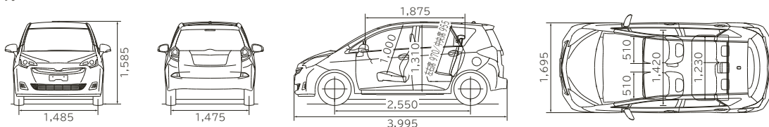
寸法図: トヨタ ラクティス 1.5G 2WD (単位:mm)
