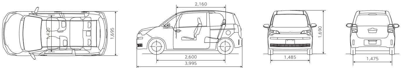
トヨタ スペイド 寸法図 F(2WD) 単位:mm
