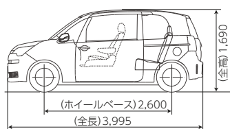
X(2WD)助手席リフトアップシート車 "Aタイプ"
