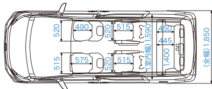
■寸法図 (単位:mm) HYBRID V "L エディション" (7人乗り・E-Four)
