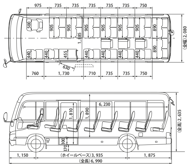
ロングボディ 26人乗りパッケージ
