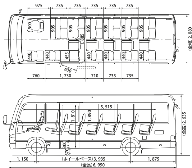
ロングボディ 24人乗り
