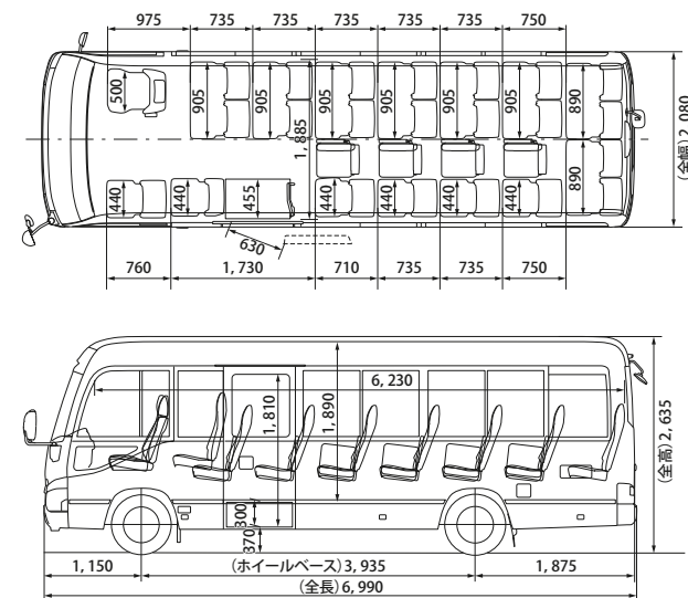
ロングボディ 27人乗りパッケージ
