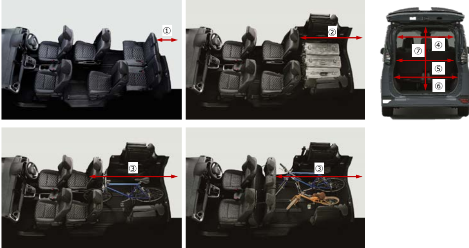
キャプテンシート (セカンドシートは背もたれが起きた状態のイラストですが、前倒し状態での数値になります。)
