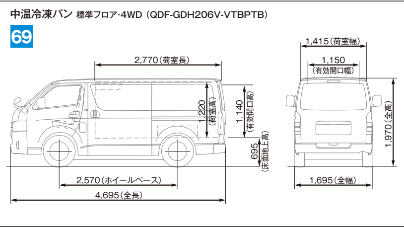
■ 寸法図 （単位:mm）
