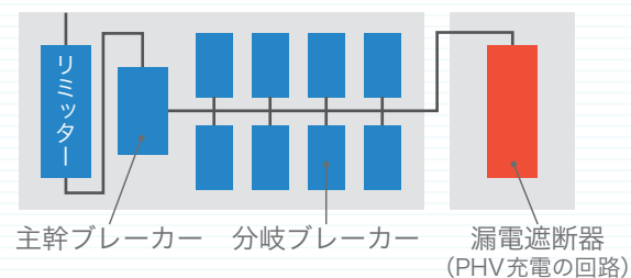
分電盤への配線例
