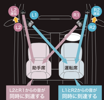
左右席同時定位原理図
