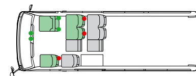
標準ボディ 9人乗り+1,250kg
