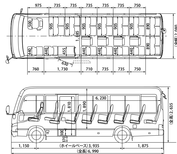
ロングボディ 27人乗りパッケージ
