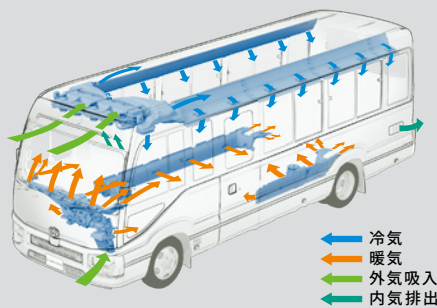
空調イメージ (リヤヒーターダクト付車)
