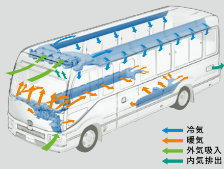
空調イメージ (リヤヒーターダクト付車)
