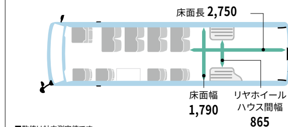
超ロングボディ 床面寸法 (単位: mm)
