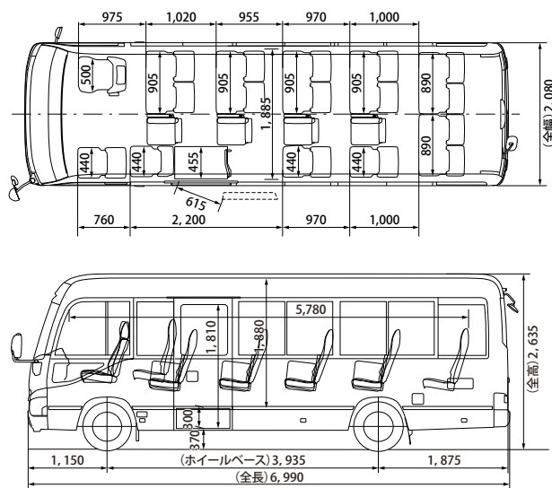
ロングボディ 21人乗り
