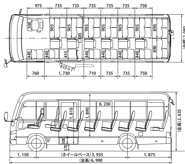
ロングボディ 29人乗り
