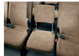
▶補助シート(はね上げ式・ シートバック上下スライド式)
