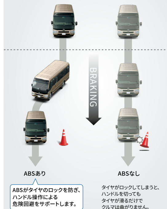
■EBD付ABS作動イメージ図
