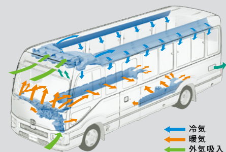
空調イメージ (リヤヒーターダクト付車)
