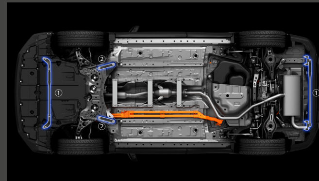
装着イメージ(①「パフォーマンスダンパー®」 ②サポートブレース)
