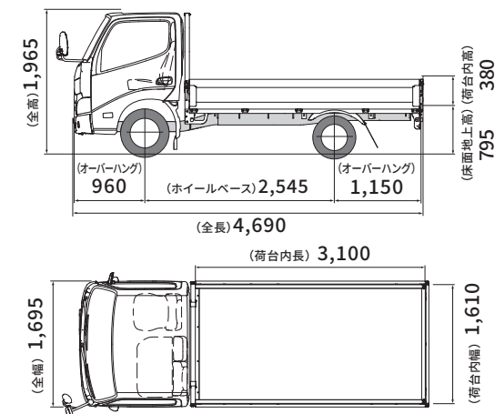
■ 寸法図 (単位:mm) 2PG-GDY281-TQMGC 車型番号 12
