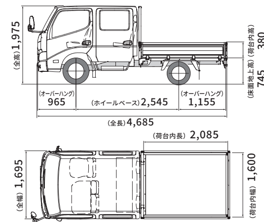
■ 寸法図 (単位:mm) 2DG-GDY281-PLTEC 車型番号 23
