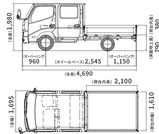
■ 寸法図 (単位:mm) 2PG-GDY231-PQMGC 車型番号 22
