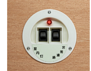
93 非常警報ブザー
