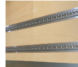
59 十字型ラッシングレール 半埋込式
