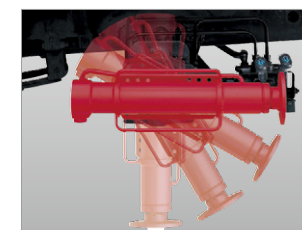
23 回転格納式リヤアウトリガ
