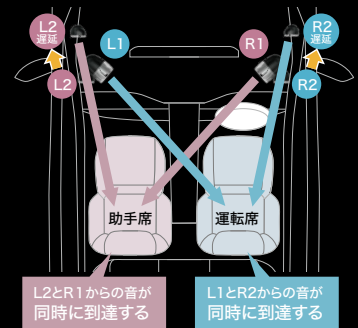
左右席同時定位原理図
