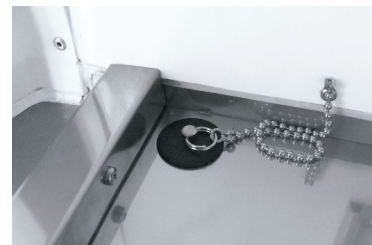
⑲ フロア後部水止め&水抜き穴追加(後左側) バックドア部に25mmの水止めを設置し、左側に水抜き穴を追加します。
