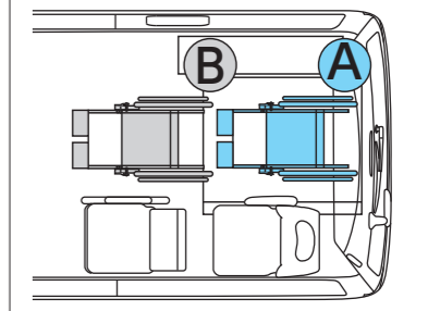
操作スイッチの装着位置 (イラストはBUタイプ)
