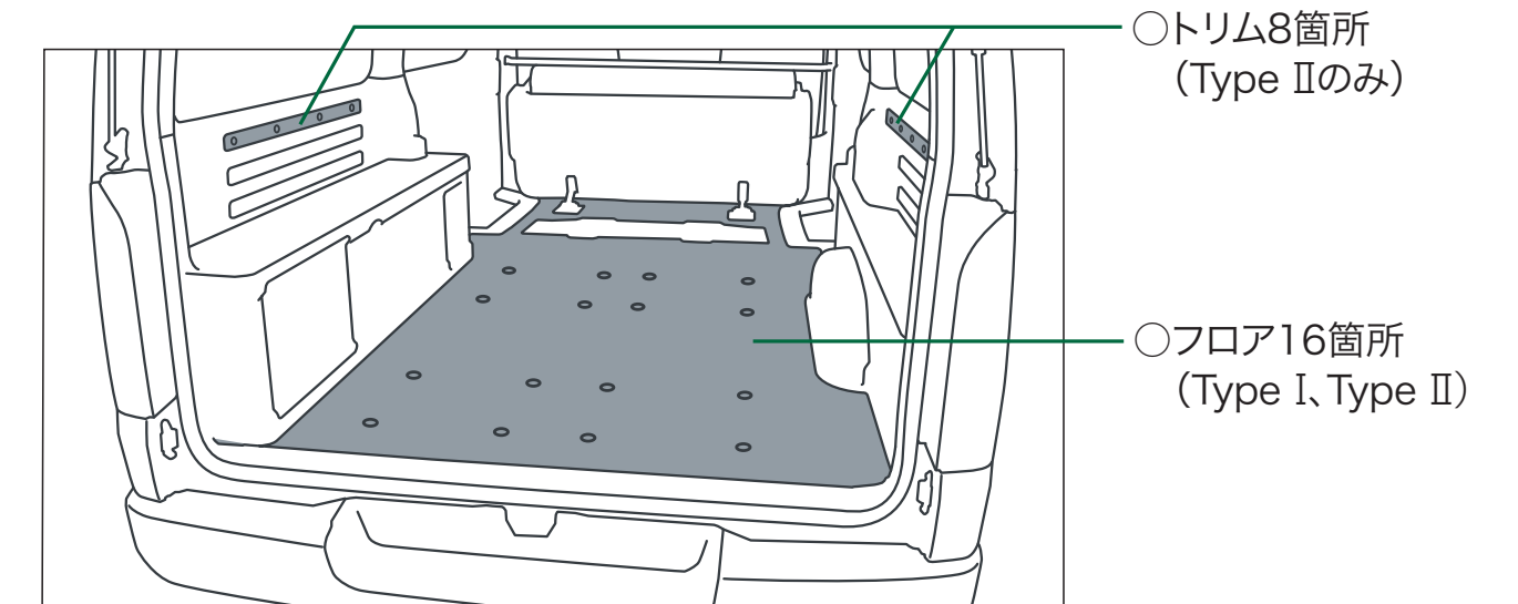
B アンカーナット位置
