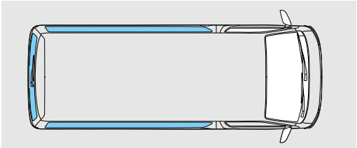
IR(赤外線)カットフィルム取付位置
