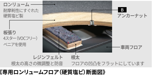
《専用ロンリウムフロア(硬質塩ビ)断面図》
