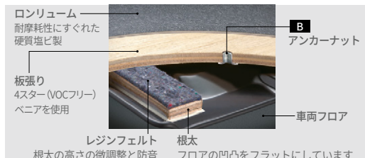
《専用ロンリウムフロア(硬質塩ビ)断面図》
