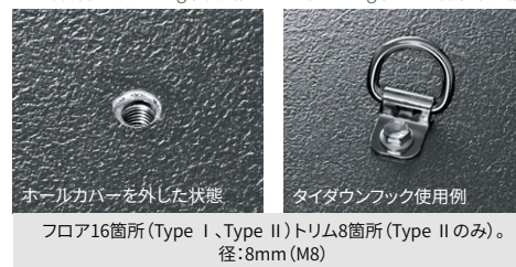
《アンカーナット位置》
