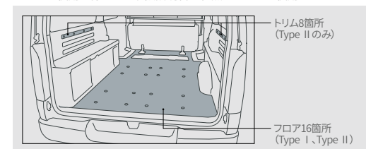
《アンカーナット位置》
