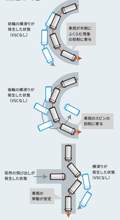
VSC作動イメージ図
