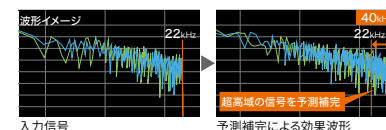
入力信号
