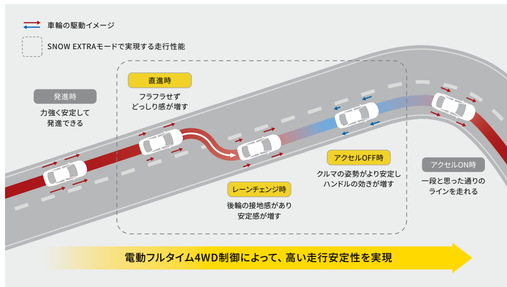
SNOW EXTRAモード制御イメージ
