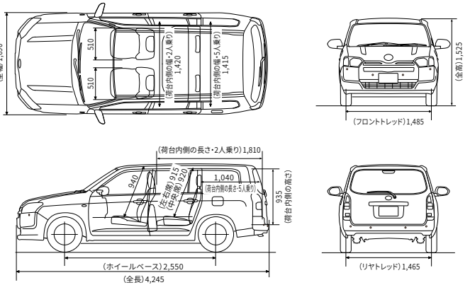
寸法図 F (ハイブリッド車) [単位: mm]
