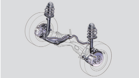
フロントサスペンション
