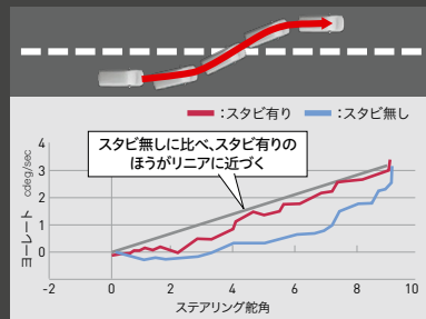
GRアスタビライザー
