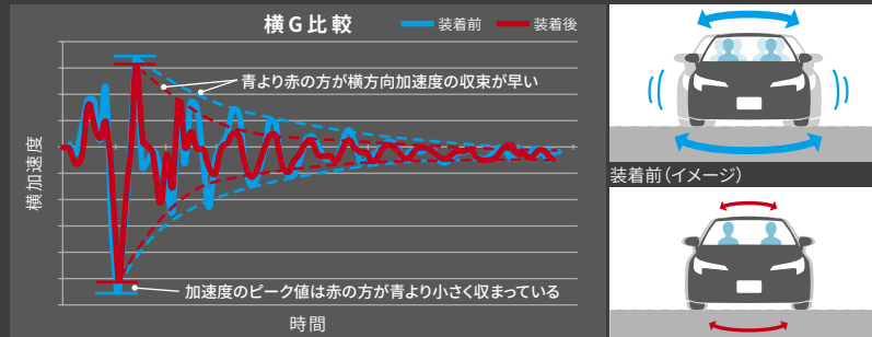
「パフォーマンスダンパー®」装着前後の横G比較データ解析 (時速20kmで30mmの段差を通過)
