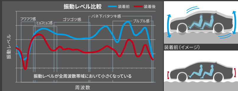
「パフォーマンスダンパー®」装着前後の上下G比較データ解析 (時速30kmで30mmの段差を通過)
