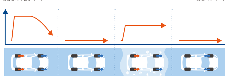
前後輪トルク配分イメージ
