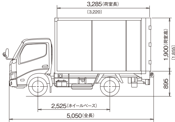
スライドリフト スマーティ TKG-XZU605-VTAGCG 車種番号 A53
