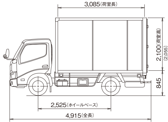
アルミバンS TKG-XZC600-VTADAG 車種番号 A1
