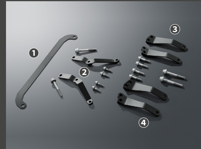
GRブレース(部品構成)
