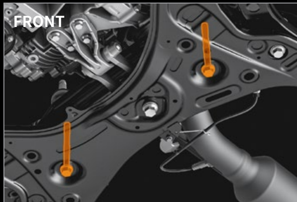
ステアリングギヤボックス x フロントサスペンションメンバー
